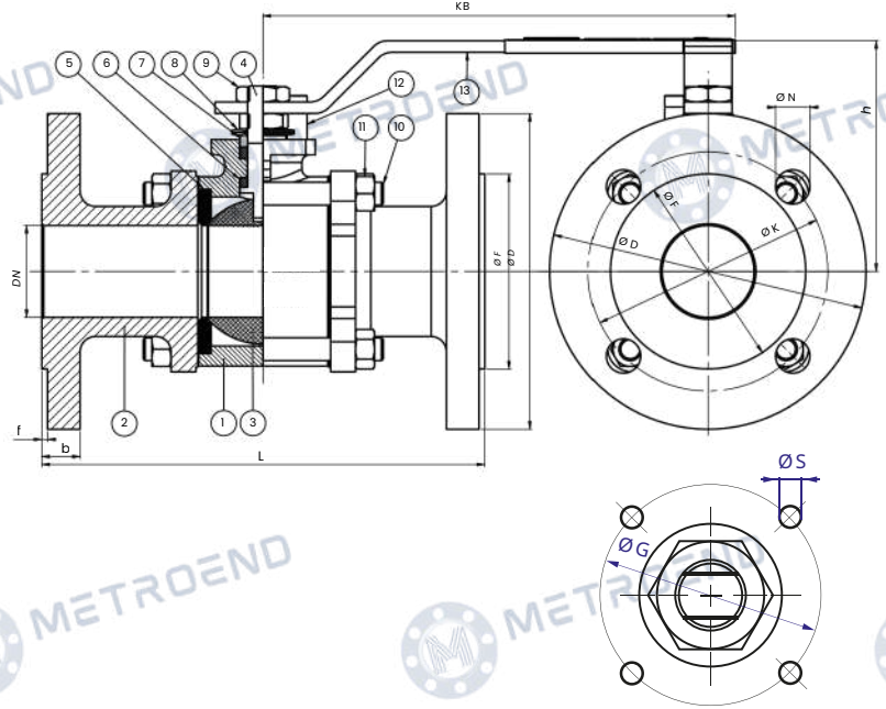
AKTÜATÖR BAĞLANTI ÖLÇÜLERİ ACTUATOR CONNECTION SIZES
